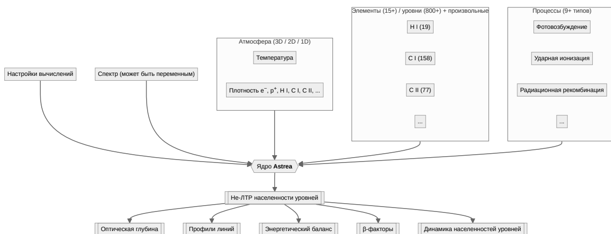
Рисунок 1: Архитектура и последовательность операций Astrea.
