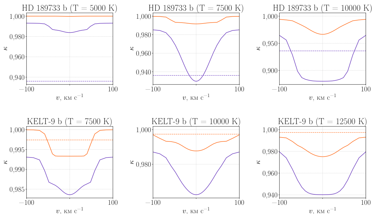
Рисунок 4: Профили поглощения линий О I 130,4 нм (■) и 777,4 нм (■) в атмосферах экзопланет HD 189733 b и KELT-9 b в зависимости от доплеровской скорости. Пунктиром обозначены результаты наблюдения глубины поглощения соответствующей линии в атмосфере соответствующей экзопланеты.
