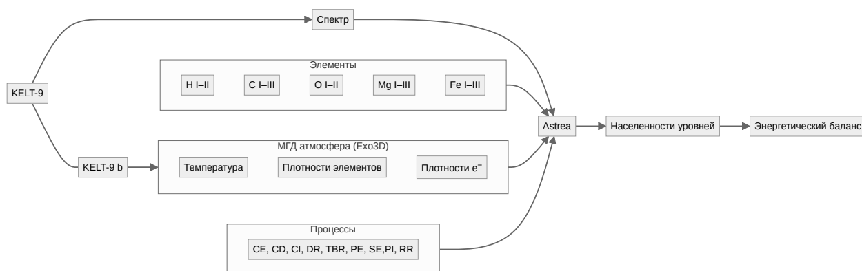
Рисунок 6: Конфигурация вычислений для исследования энергетического баланса экзопланеты KELT-9 b.
