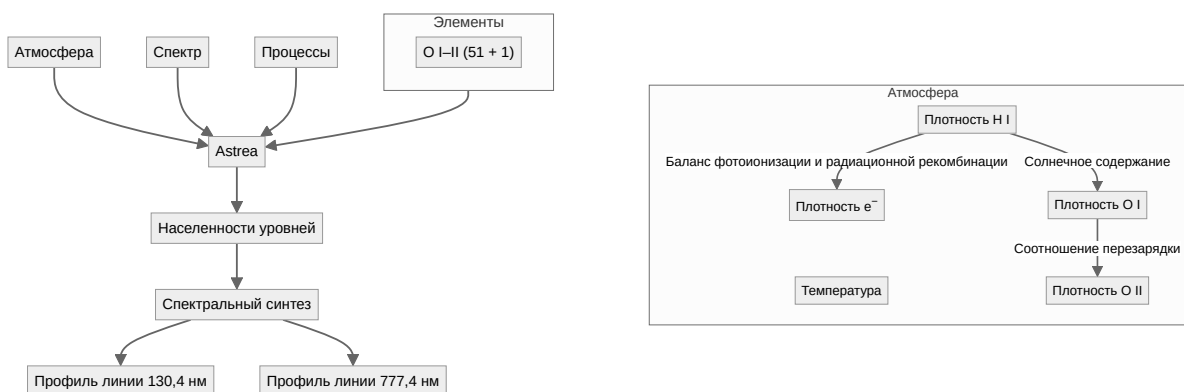
Рисунок 3: Конфигурация вычислений для исследования поглощения в линиях O I 130,4 нм и 777,4 нм.
