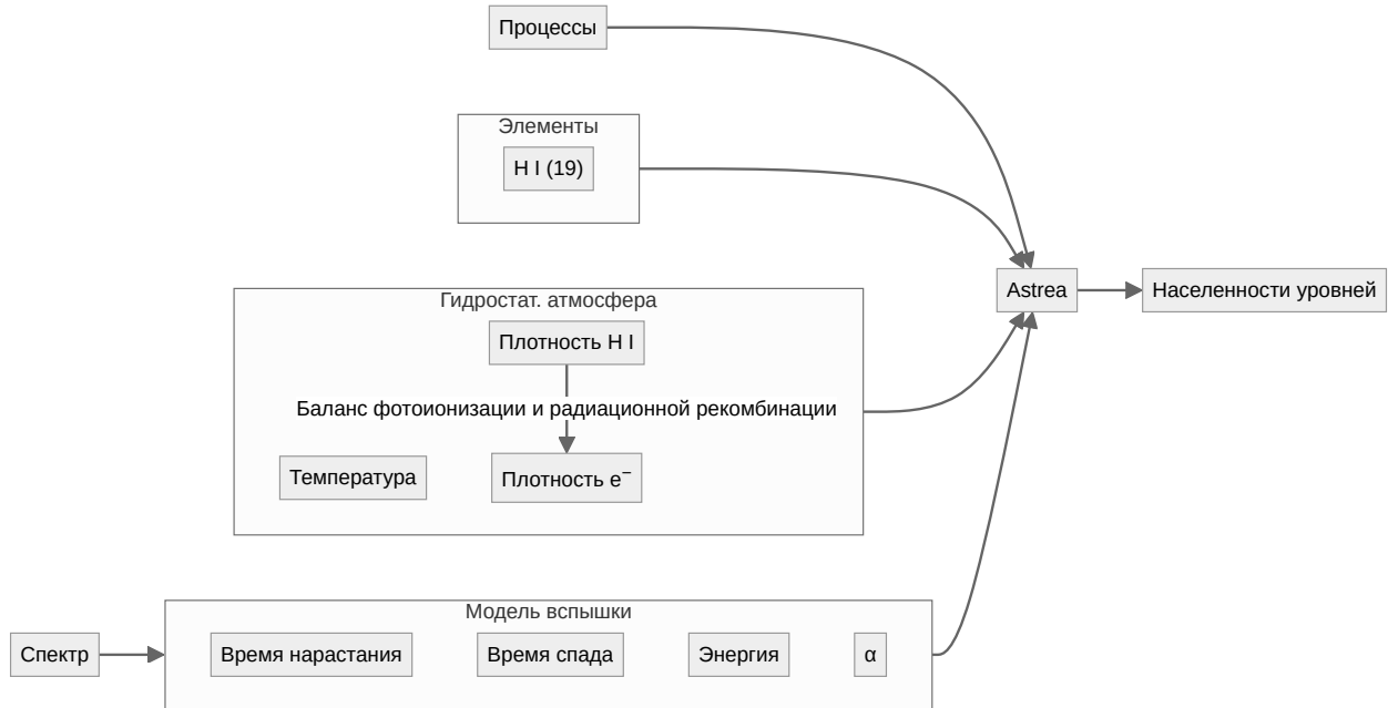
Рисунок 11: Конфигурация вычислений для исследования влияния вспышечной активности звезд на динамику населенностей уровней H I n = 2 и n = 3 , а также на поглощение в линиях Лайман-альфа и H-альфа.
