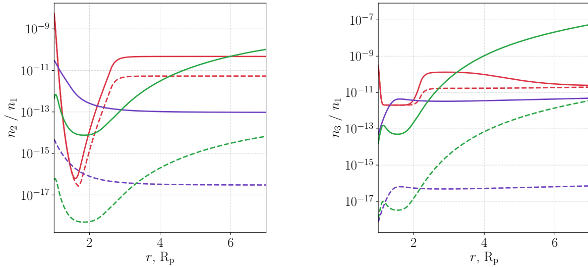
Рисунок 12: Пространственное распределение населенности уровней n = 2 и n = 3 водорода по высоте в атмосферах экзопланет KELT-9 b ( T = 6000 K, ■), TRAPPIST-1 c ( T = 500 K, ■) и HD 209458 b ( T = 3000 K, ■). Пунктирные линии соответствуют равновесным значениям до вспышки, сплошные — максимальным значениям после вспышки. Максимум достигается на 1,5\text{--}2 R_p , что обусловлено балансом фотоионизации и столкновений.
