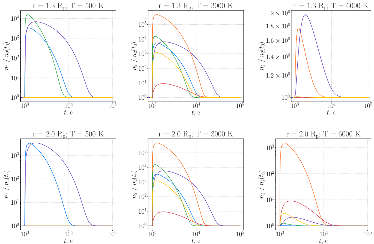
Рисунок 13: Временная эволюция отношения населенности уровня n = 2 к исходному значению до вспышки для шести экзопланетных систем при разных температурах ( T = 500 K, 3000 K и 6000 K) на высотах 1,3 R_p (характерный верхний слой) и 2 R_p (характерный разреженный слой): TRAPPIST-1 c (■), WASP-12 b (■), HD 209458 b (■), 55 Cancri e (■), KELT-9 b (■), HD 189733 b (■).
