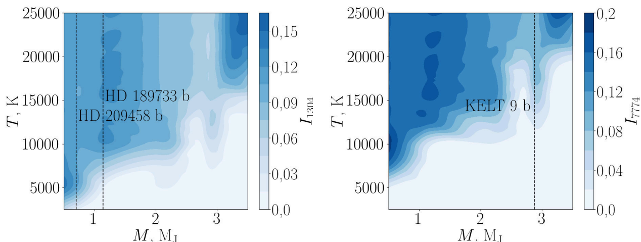
Рисунок 5: Карта обнаружения линий О I 130,4 нм и 777,4 нм в параметрическом пространстве масса—температура. Интенсивность цвета отражает глубину поглощения соответствующей линии. Важно учитывать, что эффективная температура атмосфер ультрагорячих юпитеров может достигать 10 000 К и более. Так, KELT-9 b с температурой, превышающей 10 000 К, находится в оптимальной зоне для наблюдений линии 777,4, что вполне согласуется с наблюдениями. В то же время, линия 130,4 нм обнаружима в атмосферах HD 189733 b и HD 209458 b с максимальными температурами верхних слоев до 8000 К.
