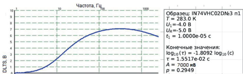
Рис. 3. Частотный скан, полученный для образца № 3 при температуре 283 К
