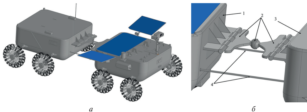
Рис. 1. Конструкция УИП ОС-8: а — общий вид; б — сцепка.
