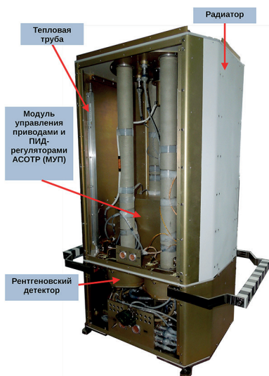
Рис. 1. Система обеспечения теплового режима СПИН-Х1-МВН
