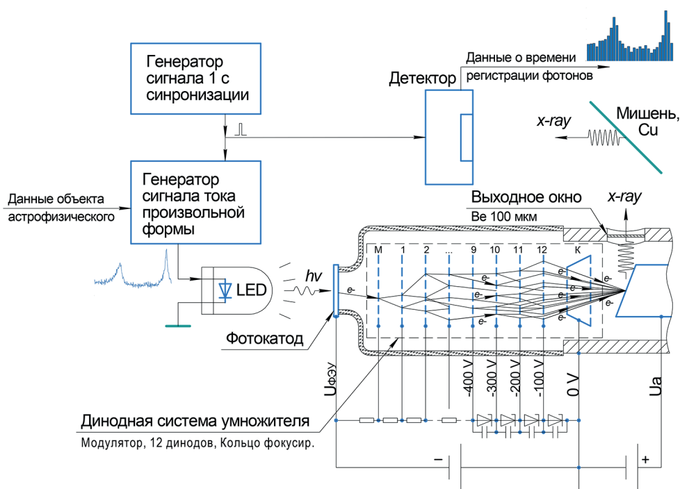
Рис. 4. Схема установки для генерации и регистрации рентгеновского излучения от флуоресцирующей мишени
