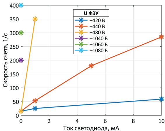
Рис. 2. Зависимость скорости счёта от тока светодиода при разном напряжении U_{\text{ФЭУ}}
