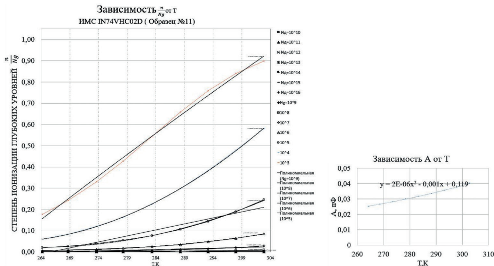
Рис. 7. Определение углов наклонов температурной зависимости амплитуды пиков DLTS-сигналов и температурных зависимостей ионизированных глубоких уровней для образца № 11
