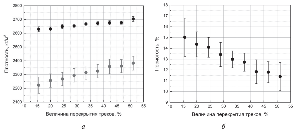
Рис. 3. Зависимости истинной (чёрные точки) и объёмной (серые точки) плотности (а) и пористости (б) образцов от величины перекрытия соседних треков. Имитатор — ГД 50–100
