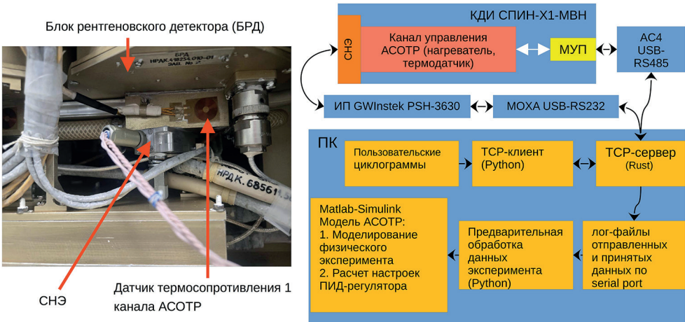
Рис. 4. ПАК испытательного стенда для КДИ СПИН-Х1-МВН
