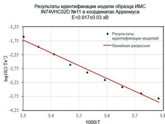
Рис. 5. Результаты идентификации модели образца № 11 в координатах Аррениуса
