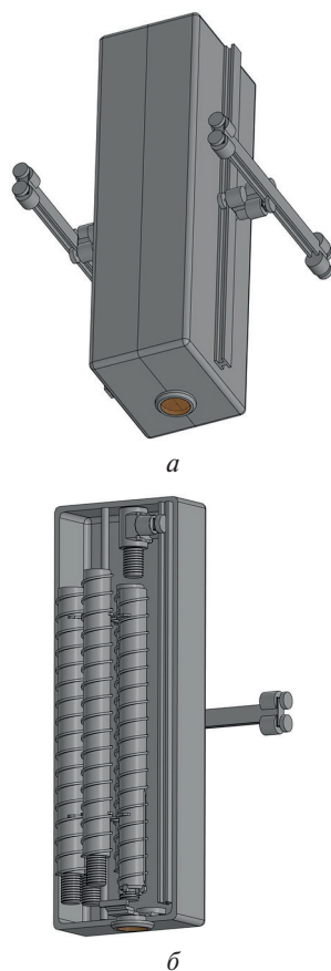
Рис. 5. ГЗУ: а — модуль с буром; б — модуль с буром в разрезе
