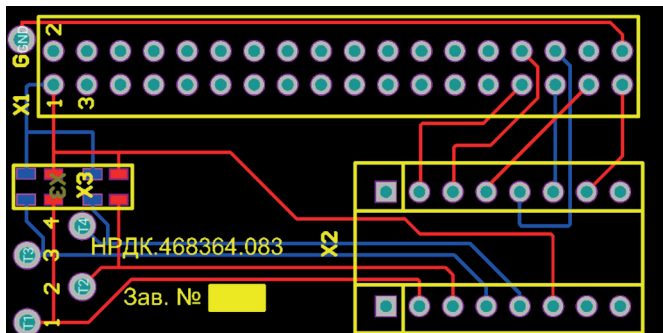
Рис. 2. Трассировка печатной платы для АЦП
