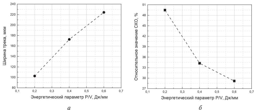
Рис. 1. Зависимости ширины (а) и среднеквадратичного отклонения ширины (б) треков, напечатанных из ГД 50–100 при толщине слоя 200 мкм.
