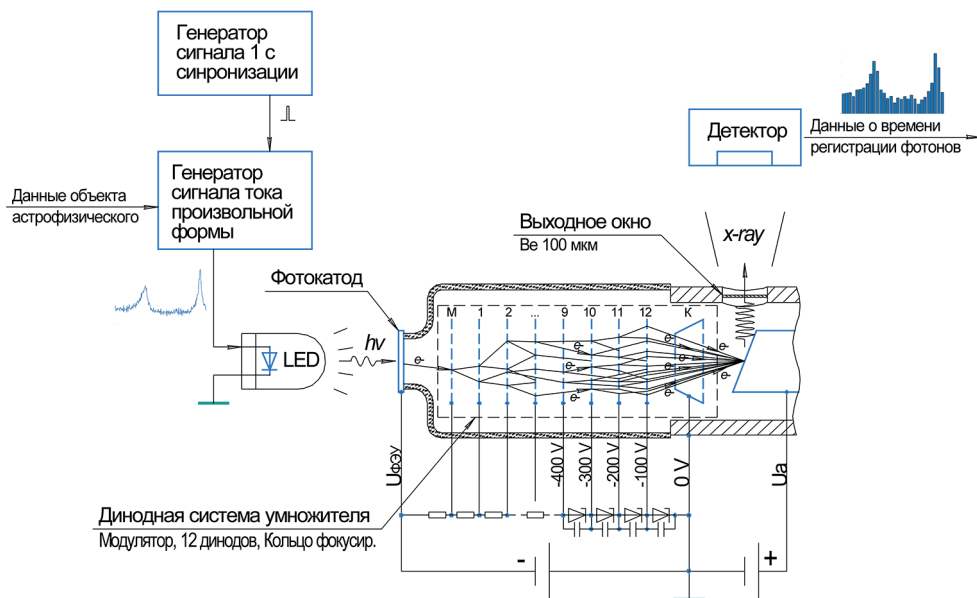
Рис. 1. Схема установки для генерации и регистрации прямого рентгеновского излучения
