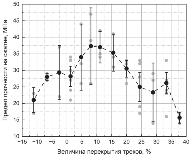
Рис. 4. Зависимость предела прочности на сжатие образцов от величины перекрытия соседних трещин: серые точки — отдельные экспериментальные данные разных образцов; чёрные точки, соединённые пунктиром, — усреднение серых точек с одинаковым перекрытием
