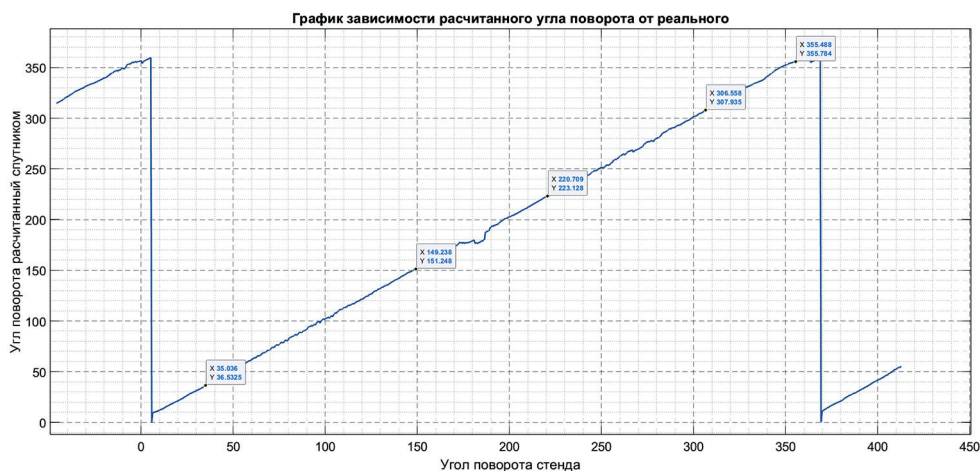
Рис. 5. Расчёт угла по алгоритму гироскопа при смене четверти
