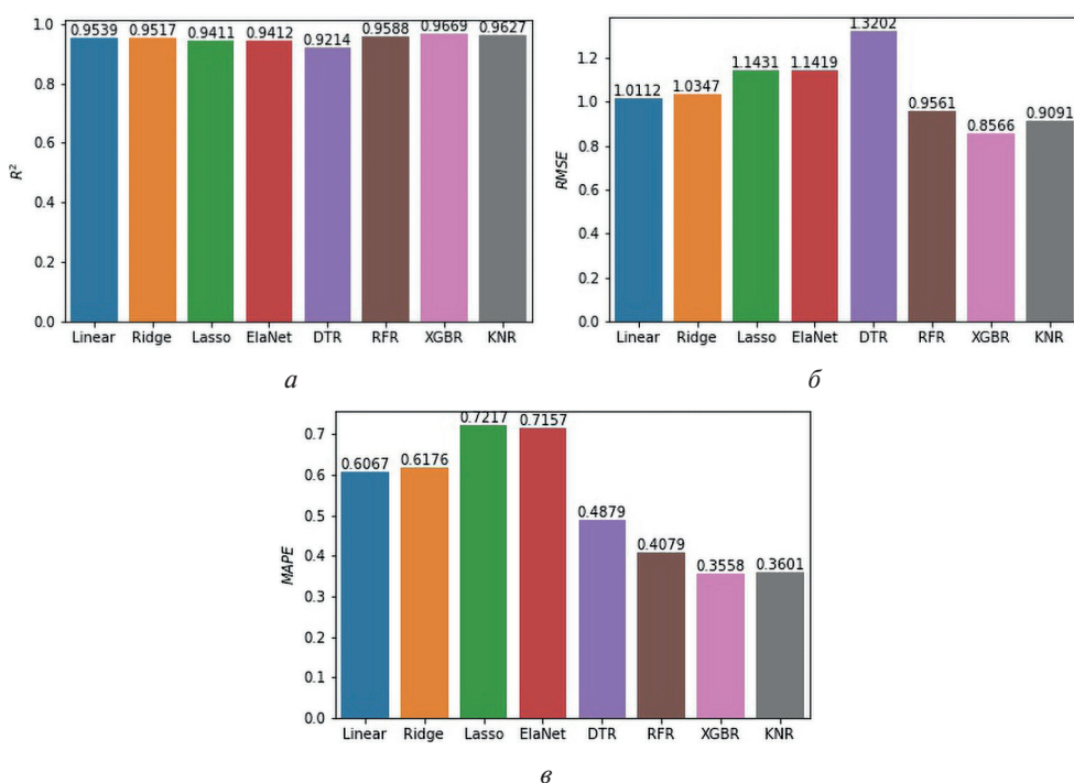
Рис. 2. Результаты метрик эффективности по данным за 2023 г.: а — R^2 ; б — RMSE; в — MAPE
