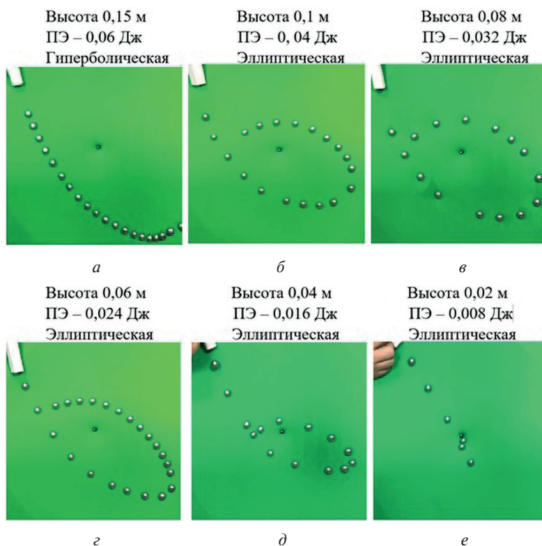
Рис. 2. Траектории полёта шарика в зависимости от высоты трубки и потенциальной энергии шарика
