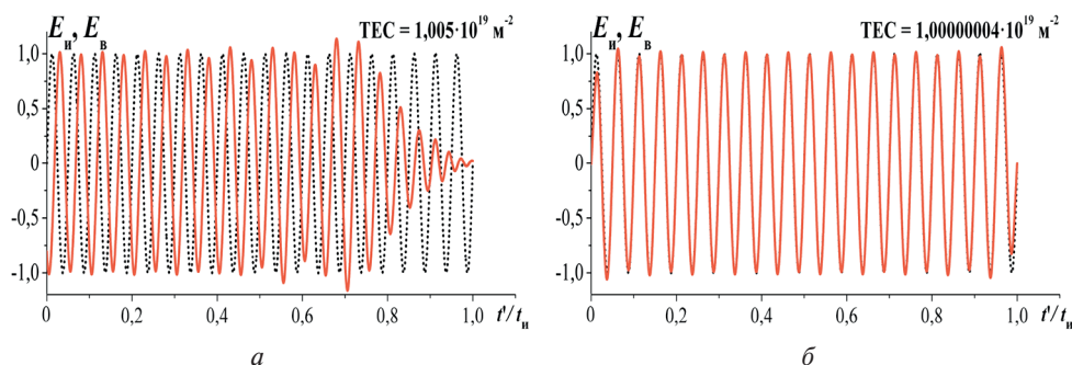
Рис. 8. Напряжённость поля восстановленного (красные кривые) и излучаемого (чёрные кривые) синусоидального импульса из рис. 3г при ТЕС = 1,005 \cdot 10^{19} \text{ м}^{-2} (а) и 1,00000004 \cdot 10^{19} \text{ м}^{-2} (б)
