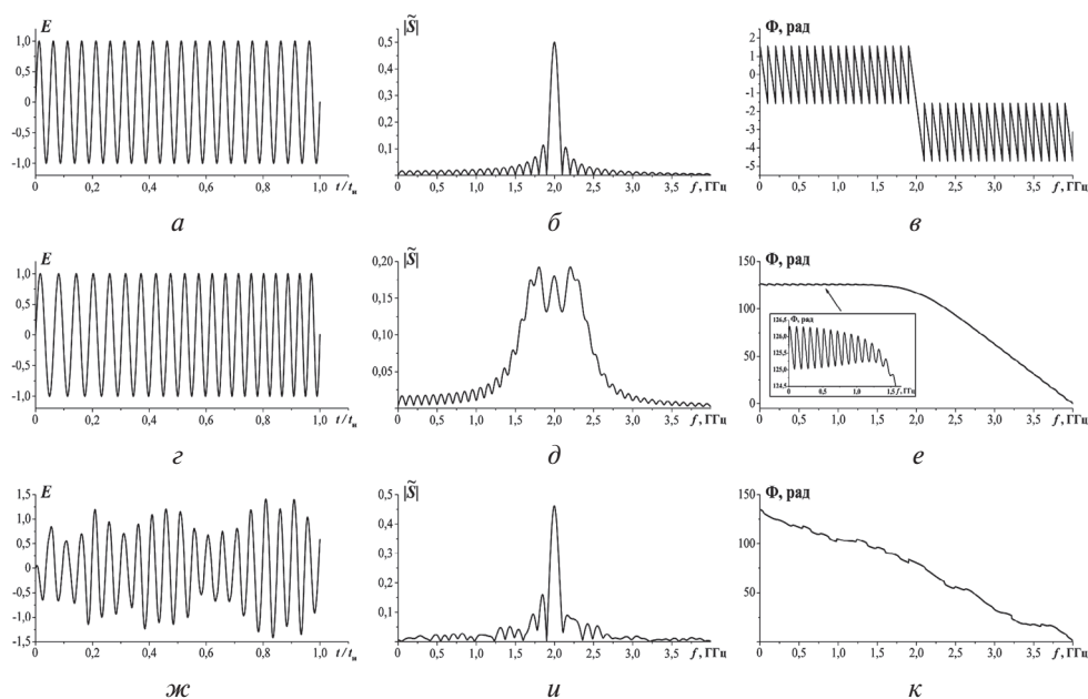
Рис. 1. Напряжённость поля (а, з, ж), амплитудные (б, д, и) и фазовые (в, е, к) спектры синусоидального (а–в); ЛЧМ (з–е) и хаотического (ж–к) радиоимпульсов при f' = 2 ГГц, t_{\text{и}} = 10 нс, \Delta f = 500 МГц, D = 0,5 , \varepsilon = 0,1 , \bar{W}_{\text{и}} = 0,5
