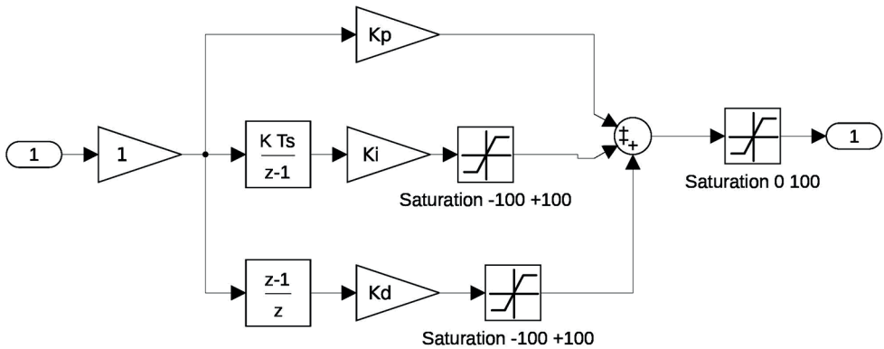
Рис. 3. Блок-схема дискретного ПИД-регулятора, реализованного в МУП
