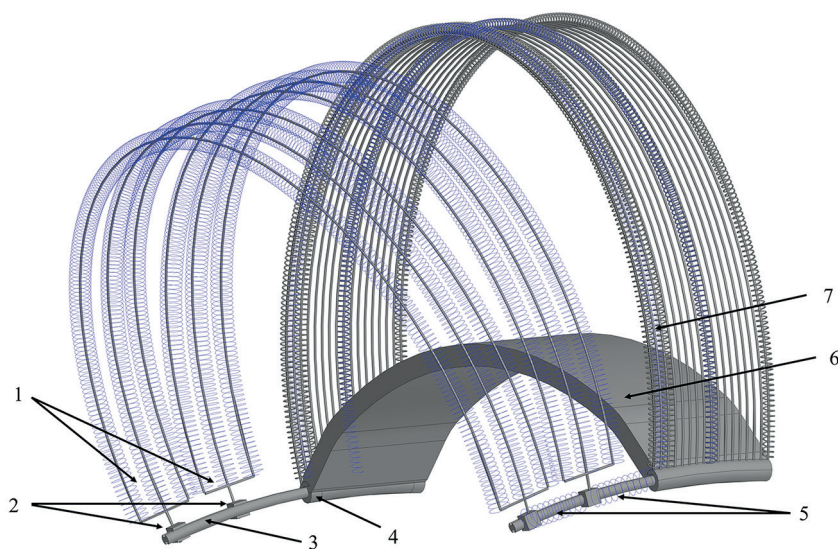
Рис. 3. Модуль бескамерной шины изменяемой жёсткости (в упрощённом виде): 1 — подвижные секции полотна; 2 — основания подвижных секций; 3 — телескопическая дуга между траками; 4 — дуга, прикреплённая к траку, в которую входит дуга 3; 5 — пружины между основаниями подвижных секций; 6 — трак; 7 — полотно неподвижной секции
