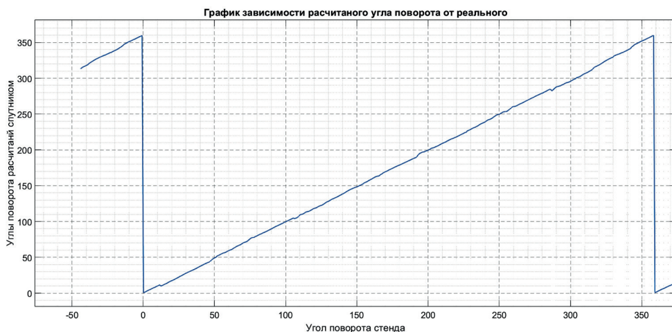
Рис. 6. Расчёт угла по алгоритму гироскопа при высокой интенсивности света
