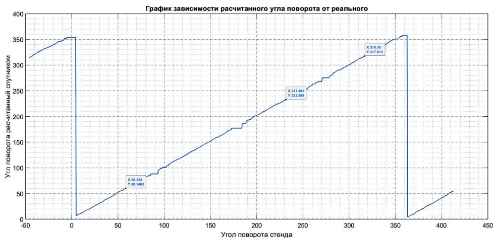
Рис. 3. Расчёт угла по алгоритму с пороговым значением в 400 лк
