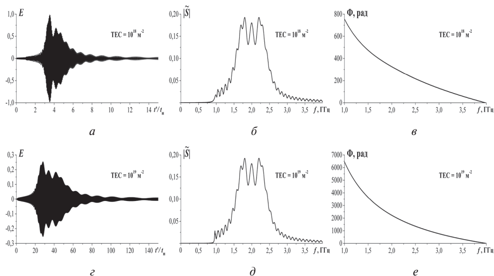
Рис. 4. То же, что и на рис. 3 для ЛЧМ радиоимпульса, изображённого на рис. 1г
