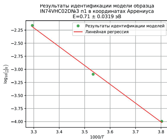
Рис. 4. Результаты идентификации модели образца № 3 в координатах Аррениуса
