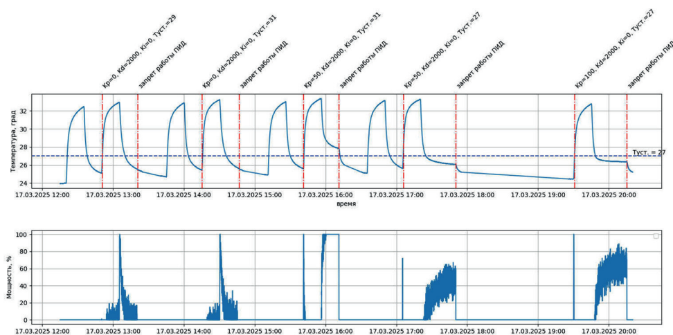
Рис. 8. Эксперименты по настройке ПИД-регулятора на 1 канале АСОТР КДИ СПИН-Х1
