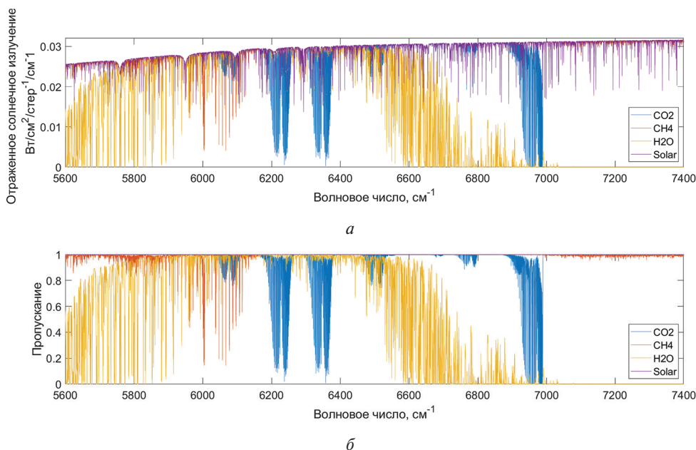
Рис. 1. Монохроматический спектр для молекул \text{CO}_2 (синяя кривая), \text{CH}_4 (красная кривая), \text{H}_2\text{O} (жёлтая кривая) и солнечный спектр (фиолетовая кривая): а — отражённого солнечного излучения; б — пропускания атмосферы
