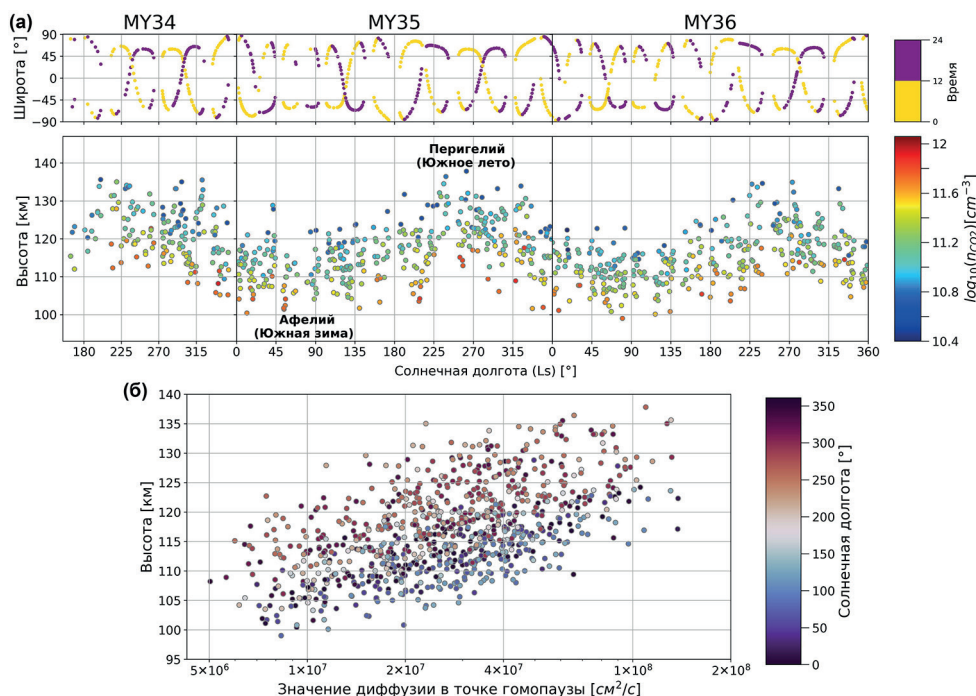
Рис. 2. Сезонное распределение высоты гомопаузы в зависимости от солнечной долготы L_s за 2,5 марсианских года (а). Цветовая шкала отражает соответствующую концентрацию \text{CO}_2 . Верхняя панель показывает широтное покрытие измерений для утреннего (охровый) и вечернего (фиолетовый) сеанса затнения. Распределение высоты гомопаузы в зависимости от значения коэффициента диффузии (б). Цветовая шкала отражает сезонную координату L_s
