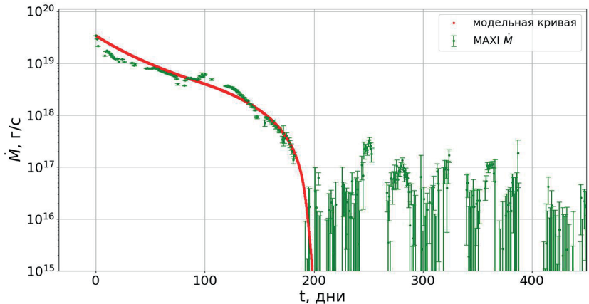
Рис. 3. Результаты моделирования всей кривой с помощью одной модели без ветра и кривая темпа аккреции, рассчитанная по данным MAXI. Параметры: \alpha = 0,81 \pm 0,04 ; C_{irr} = 0,017
