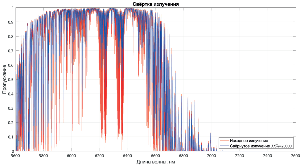
Рис. 2 Монохроматический спектр пропускания атмосферы Земли в надирной геометрии (солнечный зенитный угол равен 30^\circ ) с учётом поглощения молекул \text{CO}_2 , \text{CH}_4 , \text{H}_2\text{O} (красная кривая) и свёртка с аппаратной функцией для R = 20\,000 (синяя кривая)
