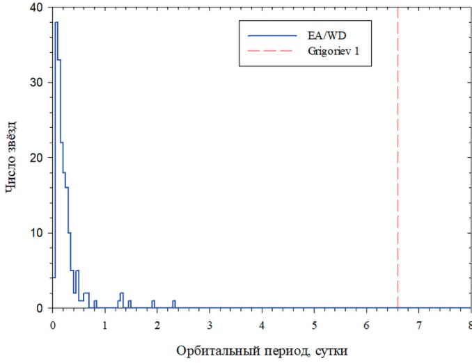
Рис. 4. Распределение 188 известных затменных переменных звёзд с белыми карликами по орбитальным периодам. Период Grigoriev 1 отмечен красной вертикальной линией
