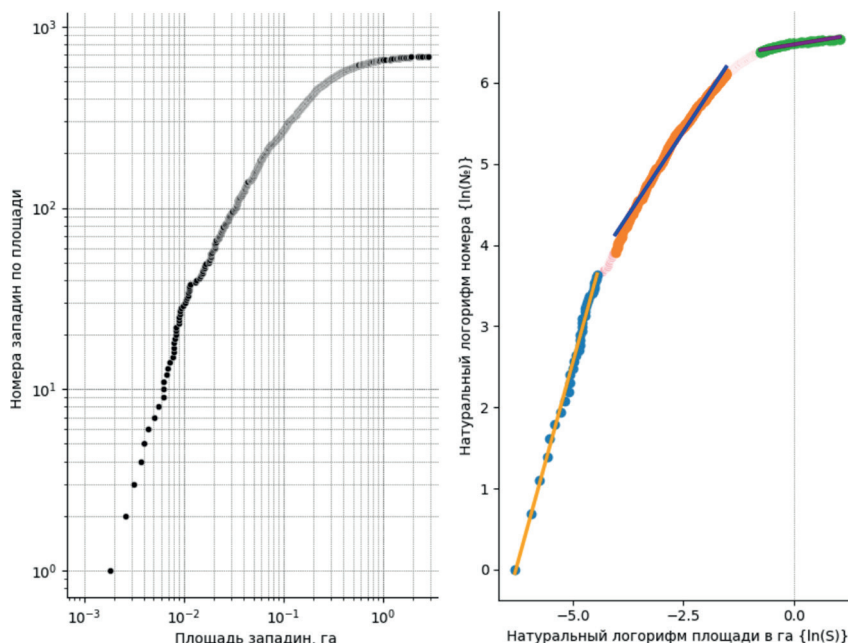
Рис. 4. Ранговый анализ площадей западин с последующей аппроксимацией
