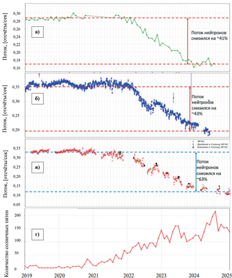
Рис. 2. Временные профили потока нейтронов: а — детектор MD эксперимента БТН-М1/МКС; б — детектор MD эксперимента ХЕНД/«Марс Одиссей»; в — детектор SFN эксперимента МГНС/«БеппиКолумбо». Временной профиль количества солнечных пятен (солнечная активность) ( г )
