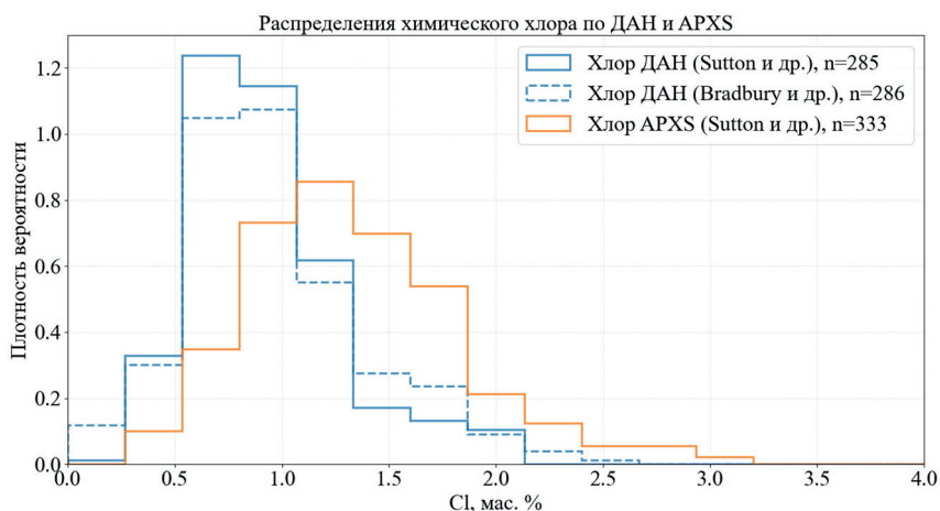
Рис. 3. Распределение химического хлора по ДАН и APXS в геологических областях: Sutton Island, Blunts Point, Pettegrove Point, Jura, Knockfarril Hill (сплошные линии) и распределение химического хлора по ДАН в Brudbury, Pahrump Hills, Hartmann's Valley и Karasburg (пунктирная линия)
