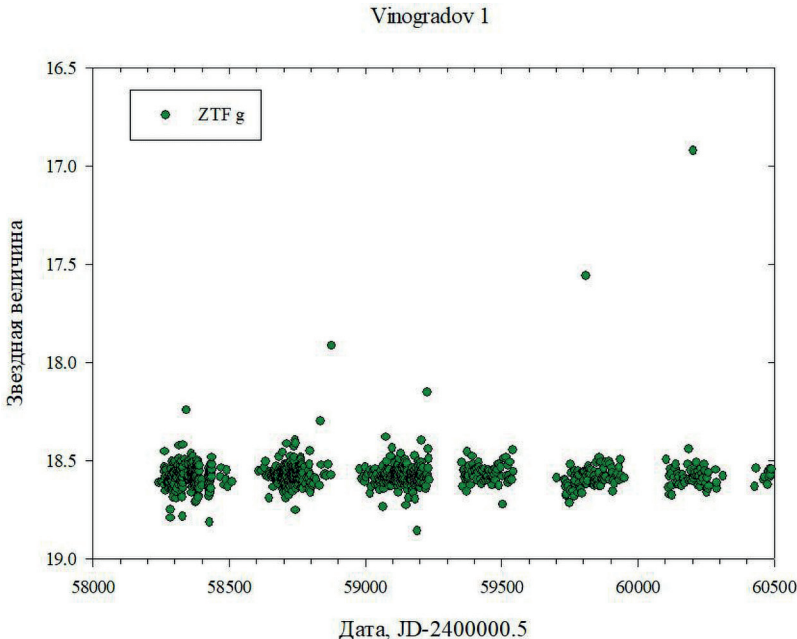
Рис. 1. Кривая блеска переменной звезды Vinogradov 1 по данным проекта ZTF
