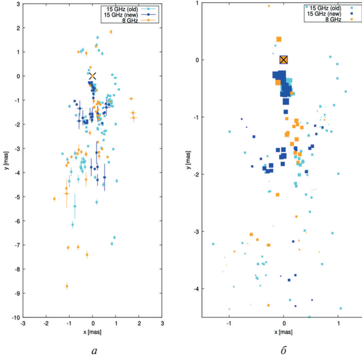
Рис. 1. Все радиокомпоненты, отображённые в плоскости xy . Голубым цветом показаны компоненты на частоте 15 ГГц, полученные при анализе данных до 2016 г., синим — новые данные, полученные в 2016–2023 гг. Оранжевым цветом также показаны новые данные, но на частоте 8 ГГц: a — все данные с крестами ошибок; b — увеличенный участок изображения a . Размер квадратов описывает величину плотности потока (в логарифмическом масштабе), минимальное отображённое значение — 1 Ян (Гц). Поток от самого источника на изображениях не показан, его местоположение обозначено чёрным крестом. Изображение взято из работы (Britzen et al., 2025)
