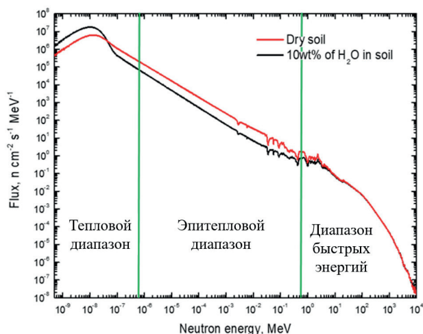
Рис. 1. Спектр нейтронов, вылетающих из реголита, характерного для горных районов Луны при различных значениях содержания водяного льда в грунте
