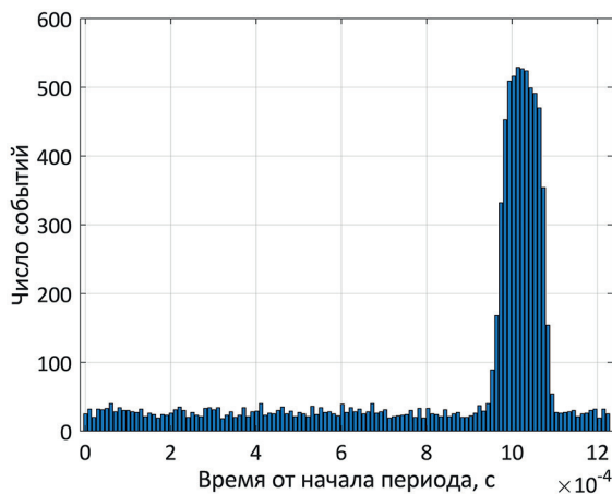
Рис. 3. Результат наложения эпох с периодом 1,234555 мс
