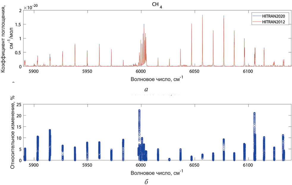
Рис. 6. Коэффициент поглощения молекулы \text{CH}_4 HITRAN2012 (красная кривая) (а) и HITRAN2020 (синяя кривая); относительное изменение коэффициента поглощения \text{CH}_4 для сильных линий (в %) (б)
