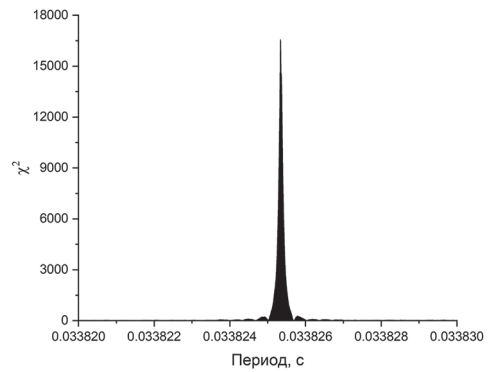
Рис. 4. Зависимость критерия Пирсона от пробного периода для данных с телескопа
