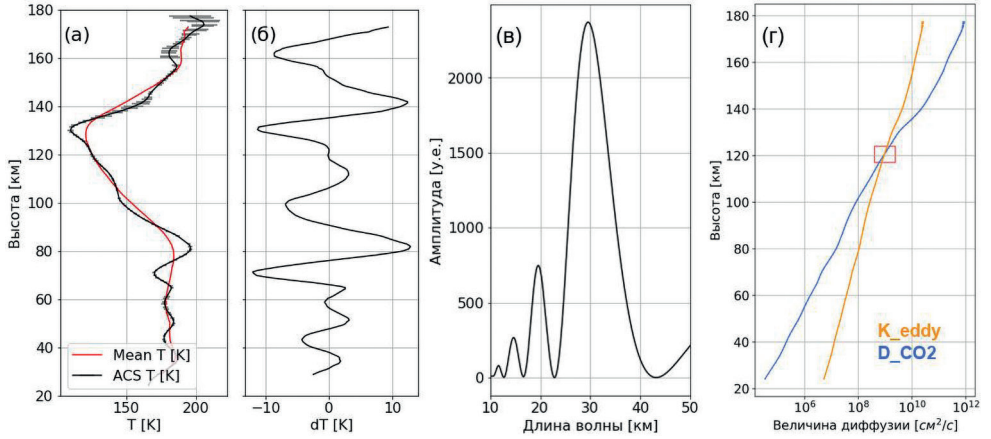
Рис. 1. Пример высотного профиля температуры T (чёрная линия с погрешностями) и усреднённый профиль температуры T_{\text{mean}} (красная линия) по данным ACS (а). Вертикальный профиль атмосферной гравитационной волны ( dT = T - T_{\text{mean}} ) (б). Пример периодограммы профиля dT в пересчёте на длину вертикальных волн (в). Пример высотных профилей турбулентной ( K_{\text{eddy}} ) и молекулярной ( D_{\text{CO}_2} ) диффузий с пересечением в области гомопаузы (с погрешностями) (г)
