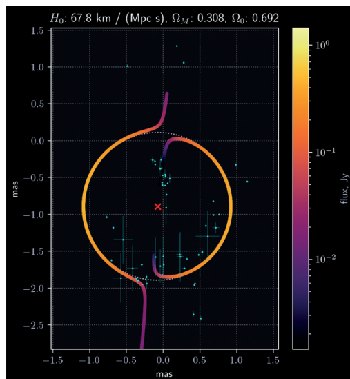
Рис. 5. Изображение модели, соответствующей лучшему набору параметров для линзы, удалённой от АЯГ. Голубыми точками показаны положения радиокомпонент за 2016–2023 гг. на частоте 15 ГГц из работы (Britzen et al., 2025)
