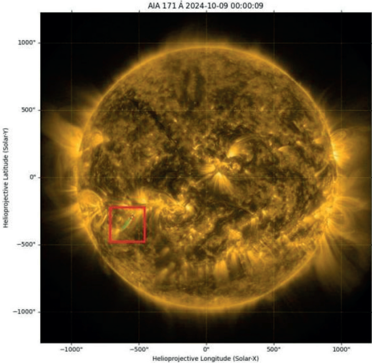
Рис. 1. Изображение с SDO/AIA, красный квадрат — наблюдаемая область, зелёного цвета — линия вдоль которой регистрируются возмущения, красный кружок — точка наблюдения, учтено вращение. Программное обеспечение — Sunpy
