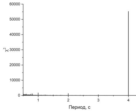
Рис. 6. Зависимость критерия Пирсона от пробного периода для сгенерированных данных с равномерным шумом для 100 тыс. событий
