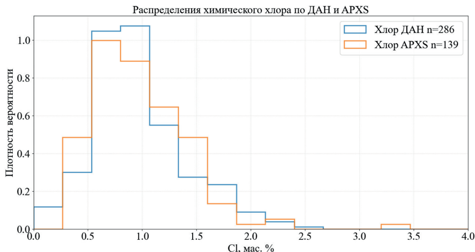
Рис. 2. Распределения химического хлора по ДАН и APXS в геологических областях: Bradbury, Pahrump Hills, Hartmann's Valley, Karasburg
