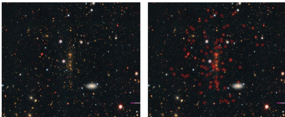
Рис. 5. Псевдоцветное изображение скопления галактик CL0238.3+2005 ( слева ), сформированное по данным обзора DESI ( англ. Dark Energy Spectroscopic Instrument) в полосах z , r , g ; красным цветом ( справа ) обведены галактики, которые принадлежат скоплению CL0238 согласно работе (Wen et al., 2024)
