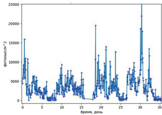
Рис. 6. Кривая блеска двойной системы Vela X-1 по данным инструмента MAXI, построенная на ограниченном участке, для демонстрации периодического движения
