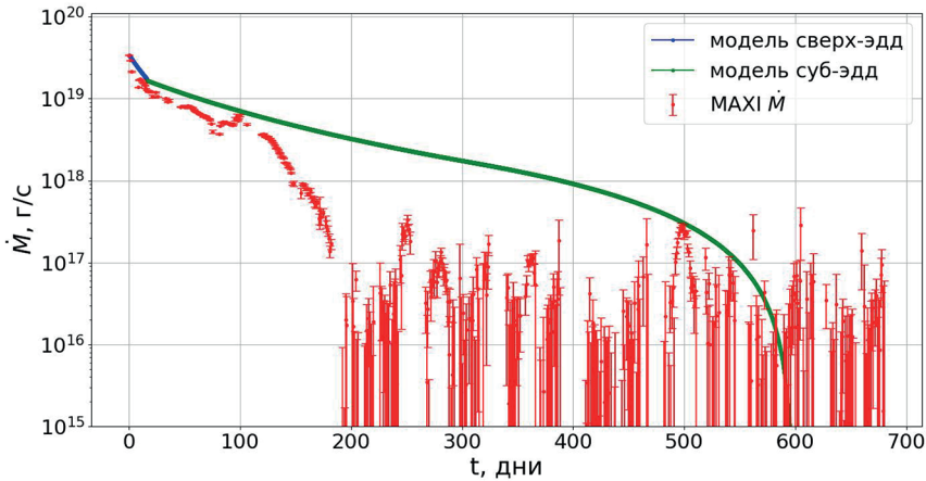
Рис. 5. Результаты моделирования с помощью двух моделей (таких же, как на рис. 4) и кривая темпа аккреции, рассчитанная по данным MAXI
