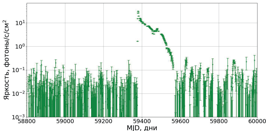
Рис. 1. Кривая блеска MAXI 4U 1543-47
