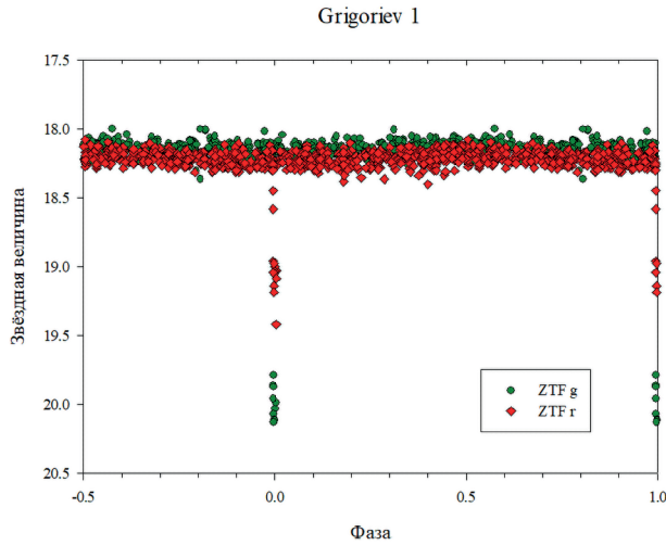
Рис. 2. Фазовая кривая блеска переменной звезды Grigoriev 1 с периодом 6,5997 сут
