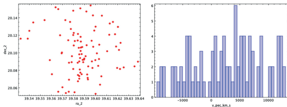
Рис. 3. Карта галактик скопления CL0238.3+2005 (слева); гистограмма скорости (справа)
