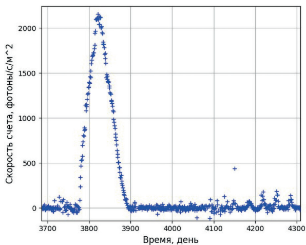
Рис. 4. Кривая блеска вспышки V 0332+53 за 2015 г.
