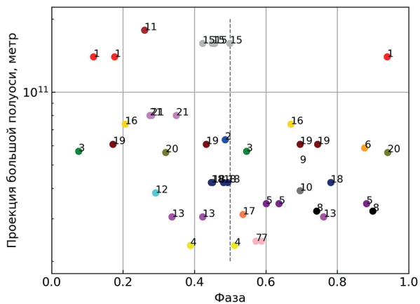
Рис. 3. Зависимость проекции большой полуоси от фазы
