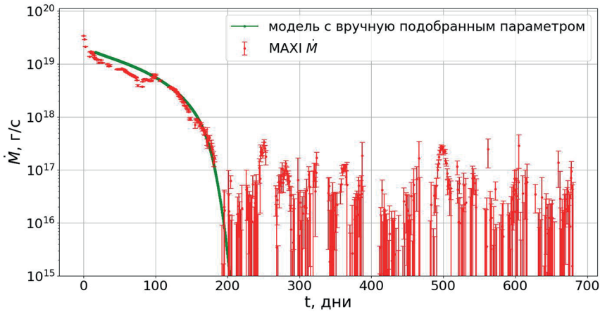
Рис. 6. Результат модели субэдингтоновской части кривой с подобранным параметром облучения C_{irr} = 0,0033 и кривая темпа аккреции, рассчитанная по данным MAXI
