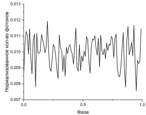
Рис. 8. Восстановленный сигнал сгенерированных данных с равномерным шумом для 100 тыс. событий для первой гармоники
