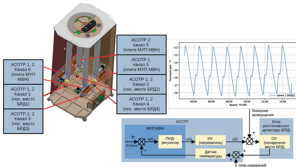
Рис. 2. Активная система обеспечения теплового режима (АСОТР) детекторов СПИН-Х
