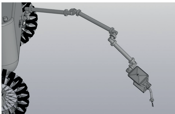
Рис. 4. Манипуляторный комплекс в разложенном положении
