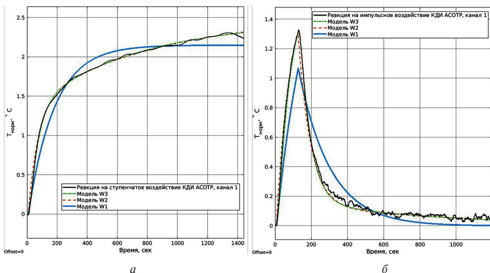
Рис. 7. Результат идентификации по отклику на ступенчатое воздействие (а) и валидация моделей по отклику на прямоугольный импульс (б)
