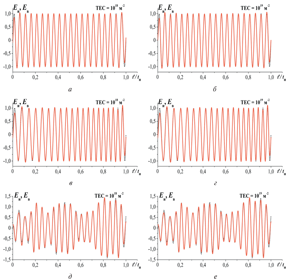
Рис. 6. Напряжённость поля восстановленного (красные кривые) и излучаемого (чёрные кривые) синусоидального ( а, б ), ЛЧМ ( в, г ) и хаотического ( д, е ) радиоимпульсов при \text{TEC} = 10^{18} \text{ м}^{-2} ( а, в, д ) и 10^{19} \text{ м}^{-2} ( б, г, е )
