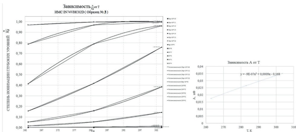
Рис. 6. Определение углов наклонов температурной зависимости амплитуд пиков DLTS-сигналов и температурных зависимостей ионизированных глубоких уровней для образца № 3
