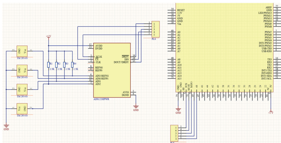
Рис. 1. Электрическая принципиальная схема переходной платы для АЦП
