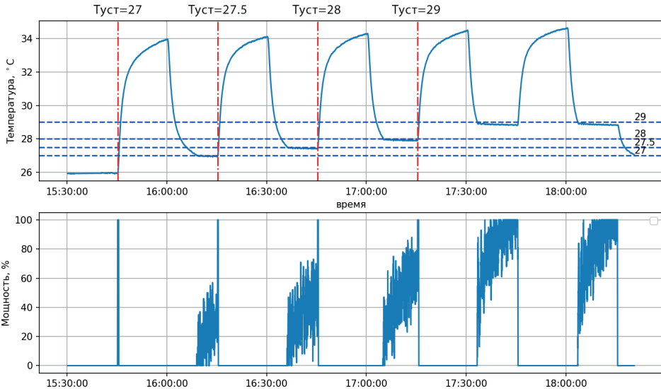
Рис. 9. Проверка работы ПИД-регулятора для канала 1 ACOTР КДИ СПИН-Х1
