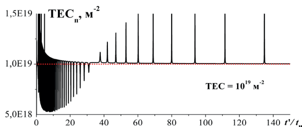
Рис. 7. Расчёт приближенного значения ТЕС трассы для синусоидального импульса из рис. 3г
