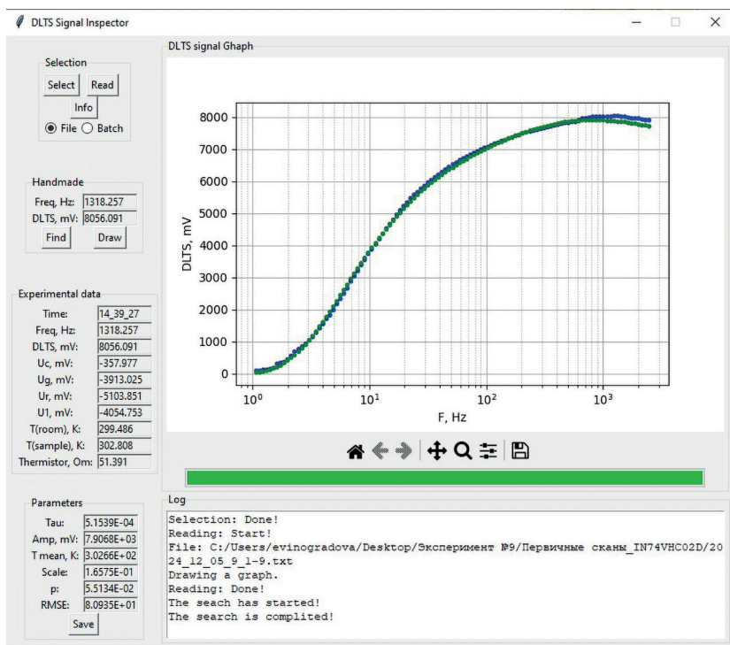
Рис. 2. Обработанный частотный скан для образца № 11 при температуре 303 К
