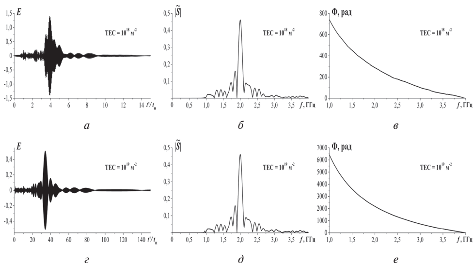
Рис. 5. То же, что и на рис. 3 для хаотического радиоимпульса, изображённого на рис. 1ж
