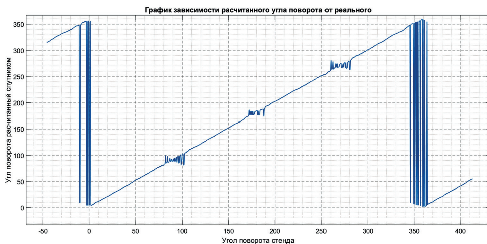
Рис. 1. Определение ориентации по начальному алгоритму
