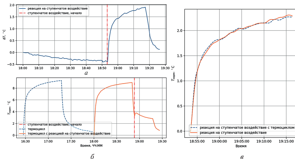
Рис. 6. Эксперимент по подаче ступенчатого воздействия на 1 канал АСОТР КДИ СПИН-Х1-МВН в условиях моделирования термоциклов
