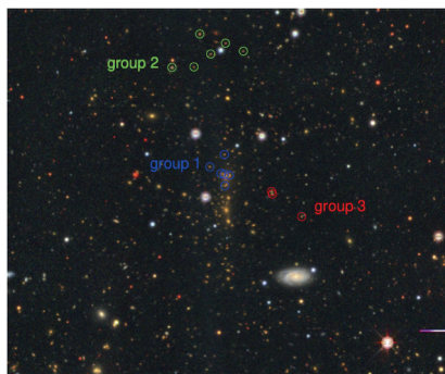
Рис. 6. Изображение скопления галактик CL0238.3+2005, где разными цветами обведены галактики, принадлежащие трём гравитационно-связанным подструктурам согласно таблице
