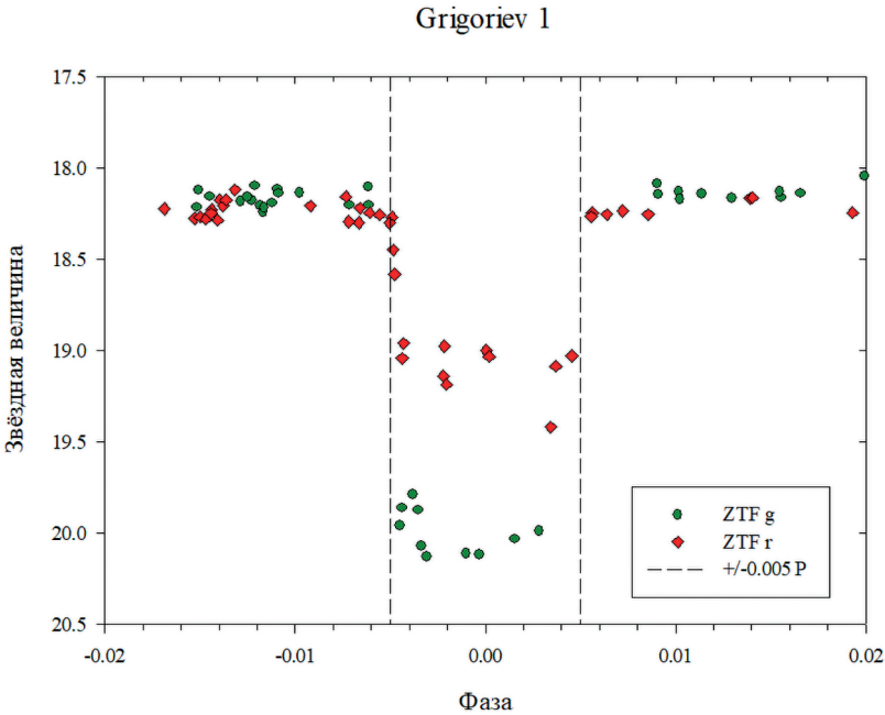
Рис. 3. Увеличенный фрагмент фазовой кривой блеска в интервале \pm 0,01 периода
