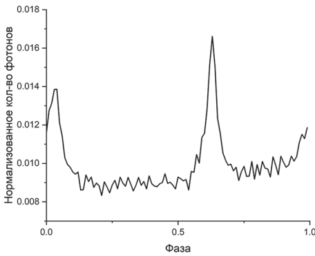
Рис. 3. Результат наложения эпох для данных с телескопа
