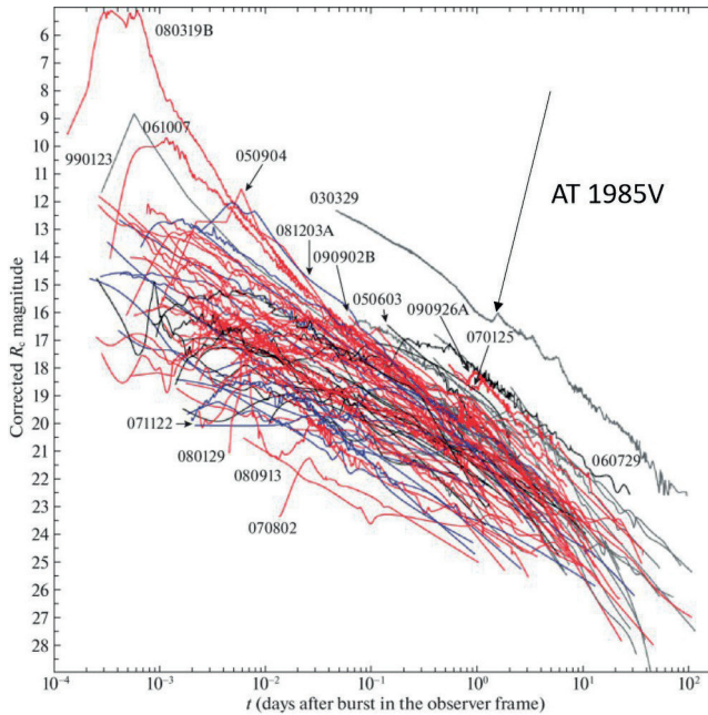
Рис. 4. Положение АТ 1985V на кривых блеска оптических послесвечений гамма-всплесков в предположении его связи с GRB 850227. По горизонтальной оси — время в сутках в логарифмической шкале, по вертикальной оси — звёздная величина в фильтре R
