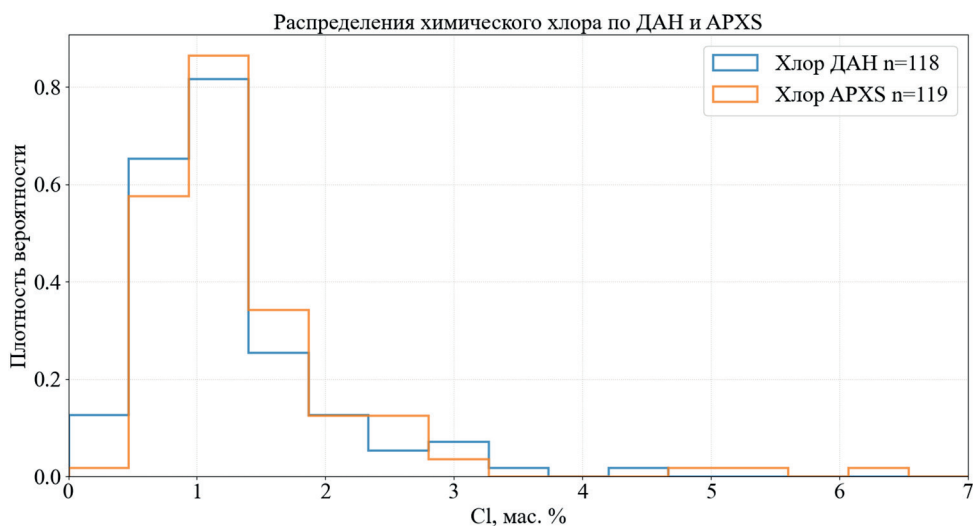
Рис. 4. Распределения химического хлора по ДАН и APXS в геологических областях: Dunnideer, Port Logan, Contigo, Catrimani
