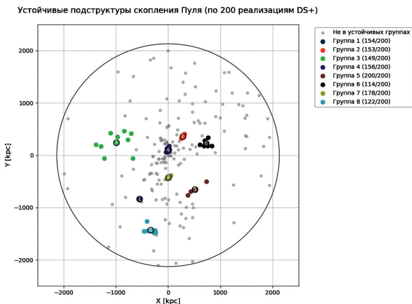
Рис. 2. Иллюстрация работы метода DS+ на скоплении Пуля. Группа 6 — Пуля. Большой серый круг иллюстрирует размер скопления и имеет радиус r_{200} = 2,13 Мпк
