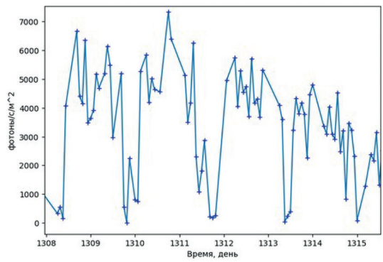
Рис. 5. Кривая блеска двойной системы Her X-1 по данным инструмента MAXI, построенная на ограниченном участке, для демонстрации периодического движения
