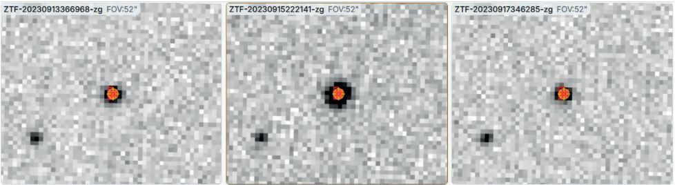
Рис. 2. Изображения звезды Vinogradov 1 в минимуме блеска и во вспышке
