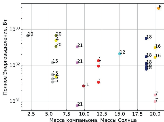
Рис. 5. Зависимость полного энергосвечения от массы компаньона
