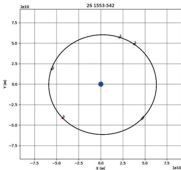
Рис. 1. Орбита 2S 1553-542
