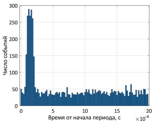
Рис. 6. Результат наложения эпох с периодом 2 мс
