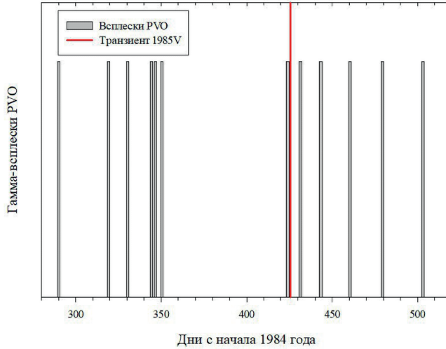
Рис. 3. Положение АТ 1985V среди гамма-всплесков, зарегистрированных PVO с сентября 1984 по май 1985 г.
