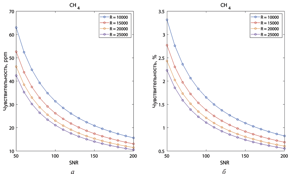
Рис. 4. Чувствительность \text{CH}_4 от соотношения сигнал-шум для R = 10\,000 (синяя кривая); 15\,000 (красная кривая); 20\,000 (жёлтая кривая); 25\,000 (фиолетовая кривая): a — в количественном виде; b — в процентном виде
