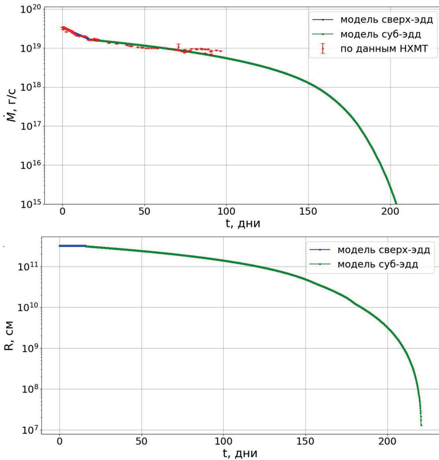
Рис. 8. Результаты финального моделирования кривой с помощью двух моделей: темп аккреции ( сверху ); эволюция внешнего радиуса горячей зоны диска ( снизу ). Параметры для модели сверхэдингтоновского участка кривой: \alpha = 1,36 ; C_{irr} = 0,0036 . Параметры для модели субэдингтоновского участка кривой: \alpha = 0,270 \pm 0,009 ; C_{irr} = 0,002546 \pm 1,4 \cdot 10^{-5}
