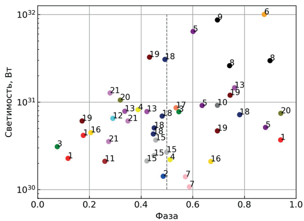
Рис. 2. Зависимость светимости от фазы
