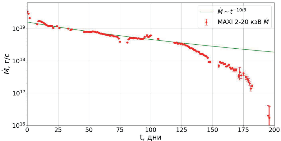
Рис. 2. Иллюстрация изменения темпа спада кривой блеска 4U 1543-47. Кривая блеска MAXI, начиная с пика вспышки, и закон изменения темпа аккреции \dot{M} \propto t^{-10/3}
