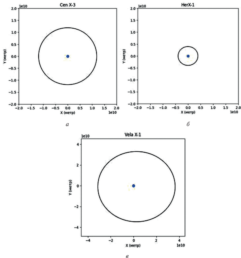
Рис. 3. Модели орбит двойных систем: a — Cen X-3; b — Her X-1; v — Vela X-1
