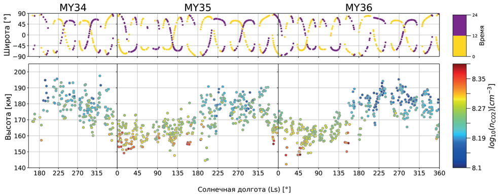
Рис. 3. Сезонное распределение высоты CO 2 экзобазы в зависимости от солнечной долготы Ls за 2,5 марсианских года. Цветовая шкала отражает соответствующую концентрацию CO 2 . Верхняя панель показывает широтное покрытие измерений для утреннего (охровый) и вечернего (фиолетовый) сеанса затмения
