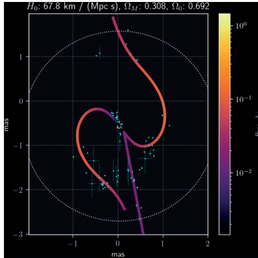
Рис. 4. Изображение модели, соответствующей лучшему набору параметров для двойной системы ЧД. Голубыми точками показано положение радиокомпонент за 2016–2023 гг. на 15 частоте ГГц из работы (Britzen et al., 2025)
