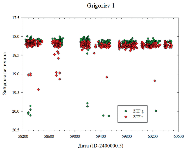
Рис. 1. Кривая блеска переменной звезды Grigoriev 1 по данным проекта ZTF. Зелёные кружки — наблюдения в фильтре g, красные ромбики — в фильтре r
