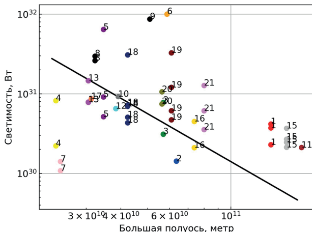
Рис. 6. Зависимость пиковой светимости от проекции большой полуоси
