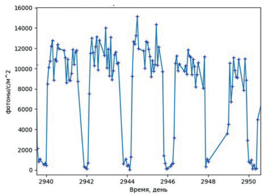
Рис. 4. Кривая блеска двойной системы Cen X-3 по данным инструмента MAXI, построенная на ограниченном участке, для демонстрации периодического движения
