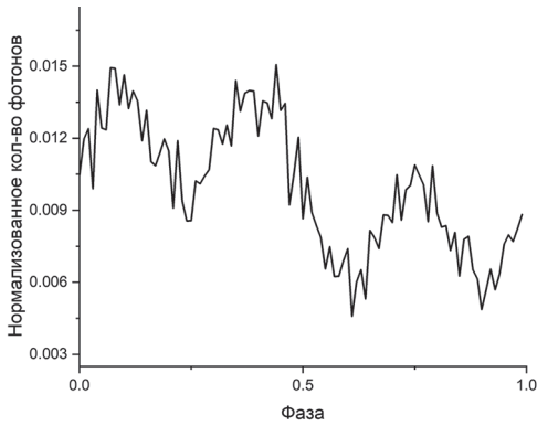
Рис. 9. Восстановленный сигнал сгенерированных данных с равномерным шумом для 100 тыс. событий для второй гармоники
