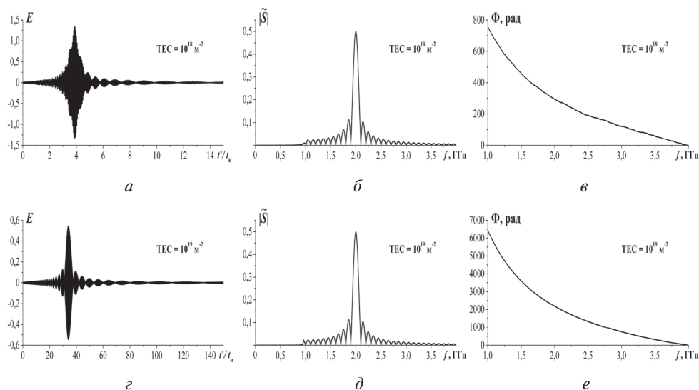
Рис. 3. Напряжённость поля (а, г), амплитудный спектр (б, д) и фазовый спектр (в, е) синусоидального радиоимпульса, изображённого на рис. 1а, в межпланетной плазме при TEC = 10^{18} \text{ м}^{-2} (а–в), 10^{19} \text{ м}^{-2} (г–е).
