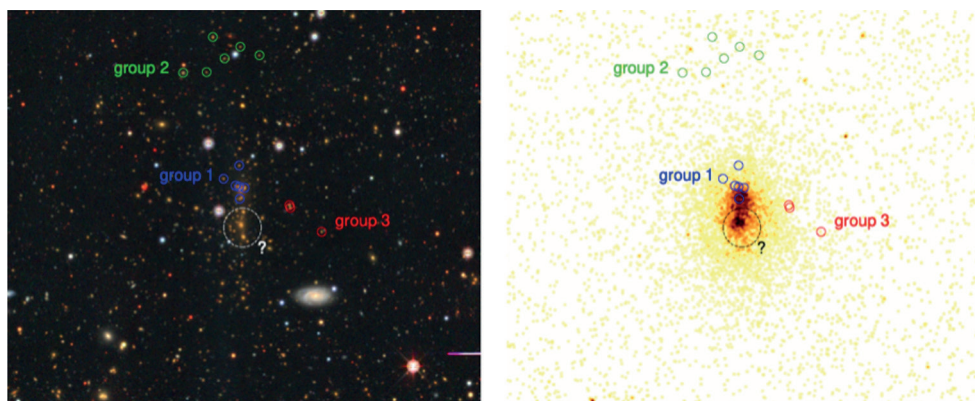
Рис. 7. Белым эллипсом обведены галактики, которые выделил бы человеческий глаз как возможную подструктуру, но алгоритм их не задетектировал ( слева ); рентгеновское изображение скопления с выделенными на основе оптического анализа подструктурами ( справа )
