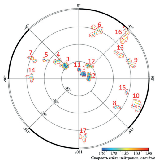
Рис. 2. Области с пониженным нейтронным потоком, найденные в результате применения метода
