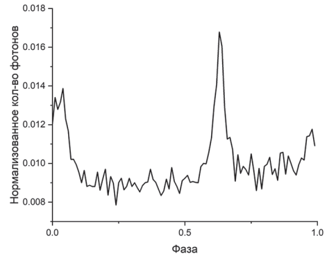
Рис. 11. Восстановленный сигнал с периодом P = 0,03382533 с
