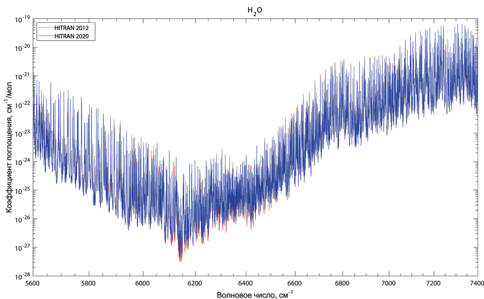
Рис. 7. Коэффициенты поглощения \text{H}_2\text{O} для HITRAN2012 (красная кривая) и HITRAN2020 (синяя кривая)
