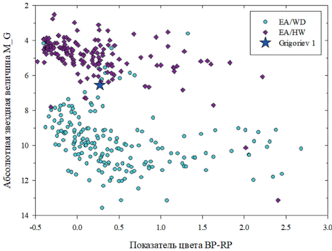
Рис. 5. Grigoriev 1 на диаграмме «цвет — светимость» для затменных переменных звёзд с белыми карликами (голубые кружки) и горячими субкарликами (фиолетовые ромбы)
