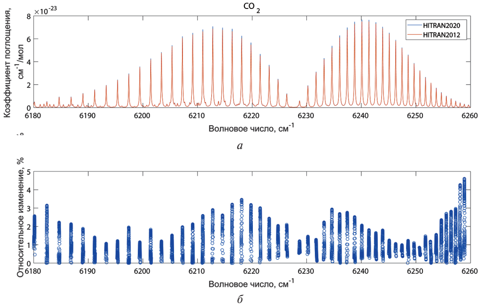
Рис. 5. Коэффициент поглощения молекулы \text{CO}_2 HITRAN2012 (красная кривая) и HITRAN2020 (синяя кривая) (а); относительное изменение коэффициента \text{CO}_2 поглощения для сильных линий (в %) (б)
