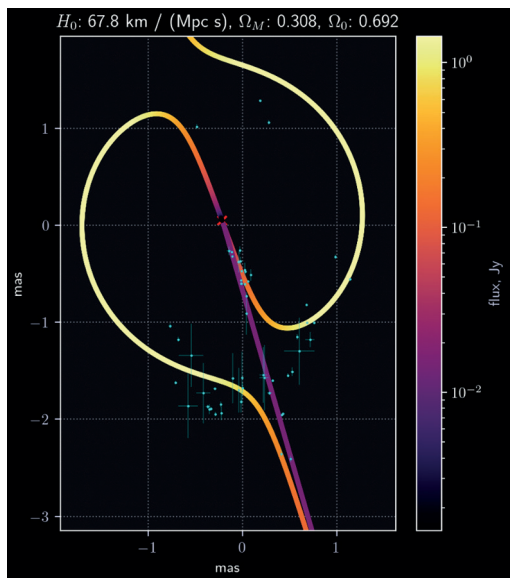
Рис. 6. Изображение модели, соответствующей лучшему набору параметров для линзирования контрджета. Голубыми точками показано положение радиокомпонент за 2016–2023 гг. на частоте 15 ГГц из работы (Britzen et al., 2025)
