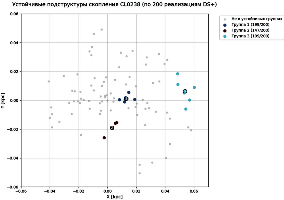
Рис. 4. Иллюстрация работы метода DS+ на скоплении CL0238.3+2005
