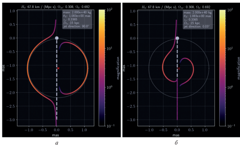
Рис. 3. Гравитационное линзирование тонкого протяжённого джета в случае, когда джет лежит в плоскости, параллельной плоскости линзы ( а ), и в случае, когда джет распространяется в сторону плоскости линзы и пересекает её ( б ). Цвет изображений характеризует значение усиления в данной точке, красным крестом отмечено положение линзы. Параметры системы подобраны так, чтобы описать наблюдения источника TXS 0506+056, т.е. красное смещение источника зафиксировано на значении z = 0,3365 , линза удалена на расстояние 15 кпк от источника, масса ЧД предполагается равной 10^{10} масс Солнца
