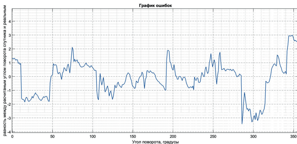
Рис. 7. Ошибка определения ориентации
