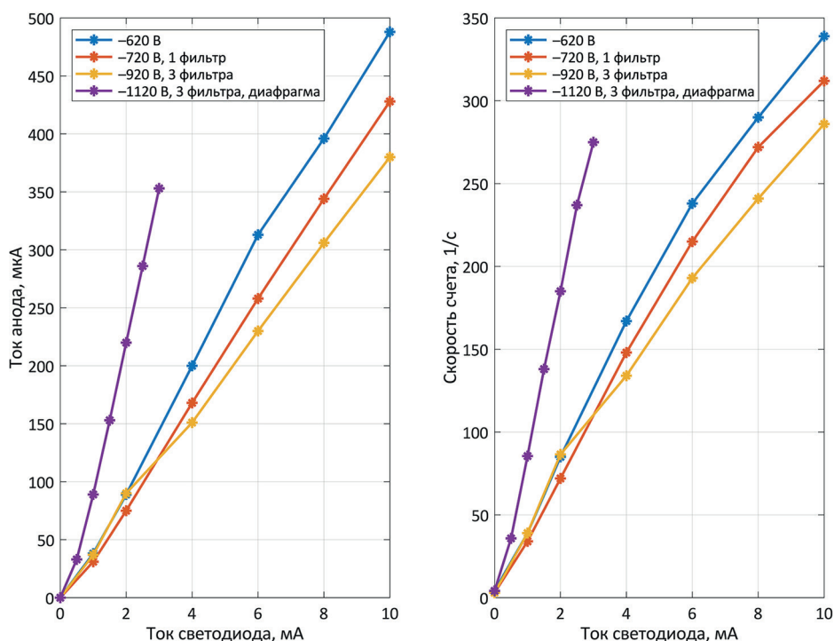
Рис. 5. Зависимости скорости счёта и тока анода от тока светодиода в экспериментах с флуоресцирующей мишенью
