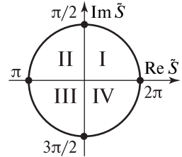
Рис. 2. Тригонометрическая окружность для расчёта фазы \Phi
