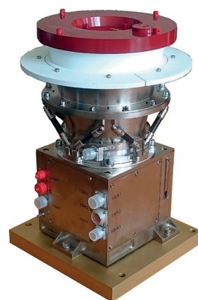
Рис. 1. Звёздный датчик ориентации повышенной точности. Внешний вид прибора
