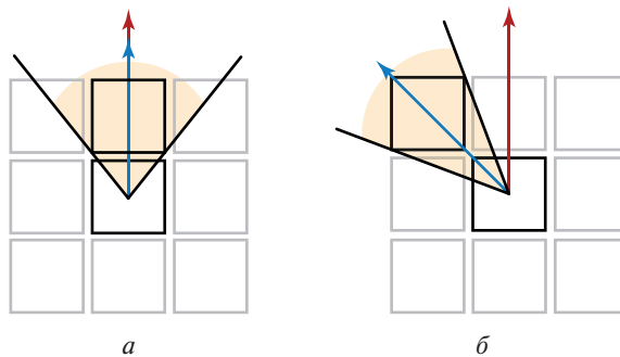
Рис. 5. Неопределённость угла рассеяния \varphi : a — при \varphi = 0^\circ ; б — при \varphi = 45^\circ
