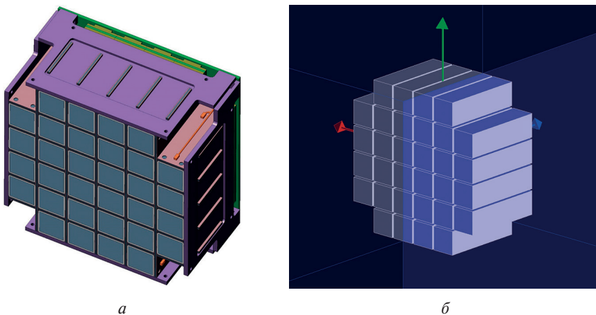
Рис. 3. Детекторная часть СГС: а — макет; б — Geant4
