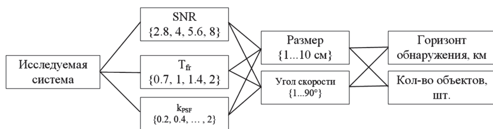
Рис. 2. Методика эксперимента
