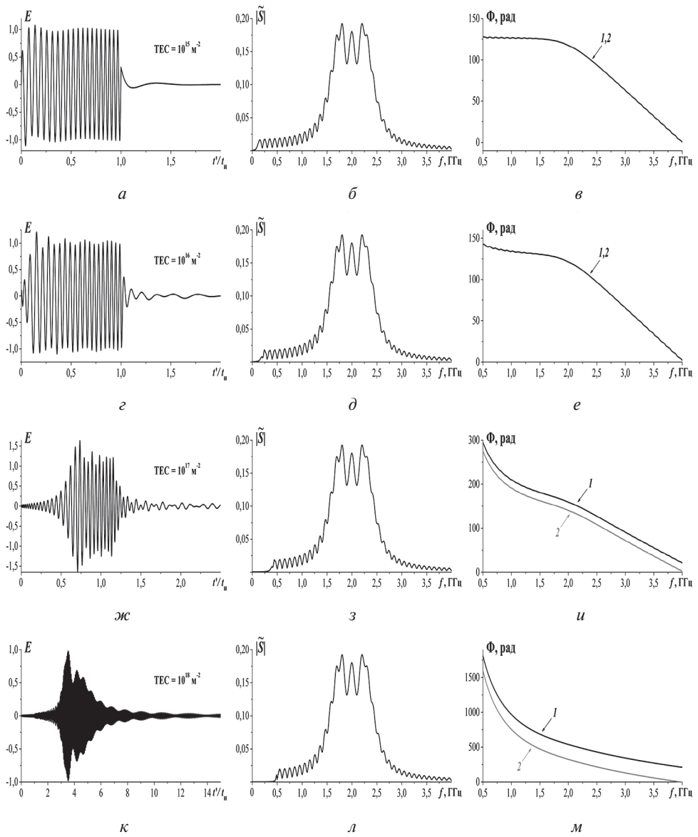
Рис. 4. То же, что и на рис. 3 для ЛЧМ радиоимпульса, изображённого на рис. 1г. \Phi = \Phi_{\text{изл}} + \Delta\Phi ( в, е, и, м кривые 1); расчёт \Phi по деформированному импульсу ( в, е, и, м кривые 2)
