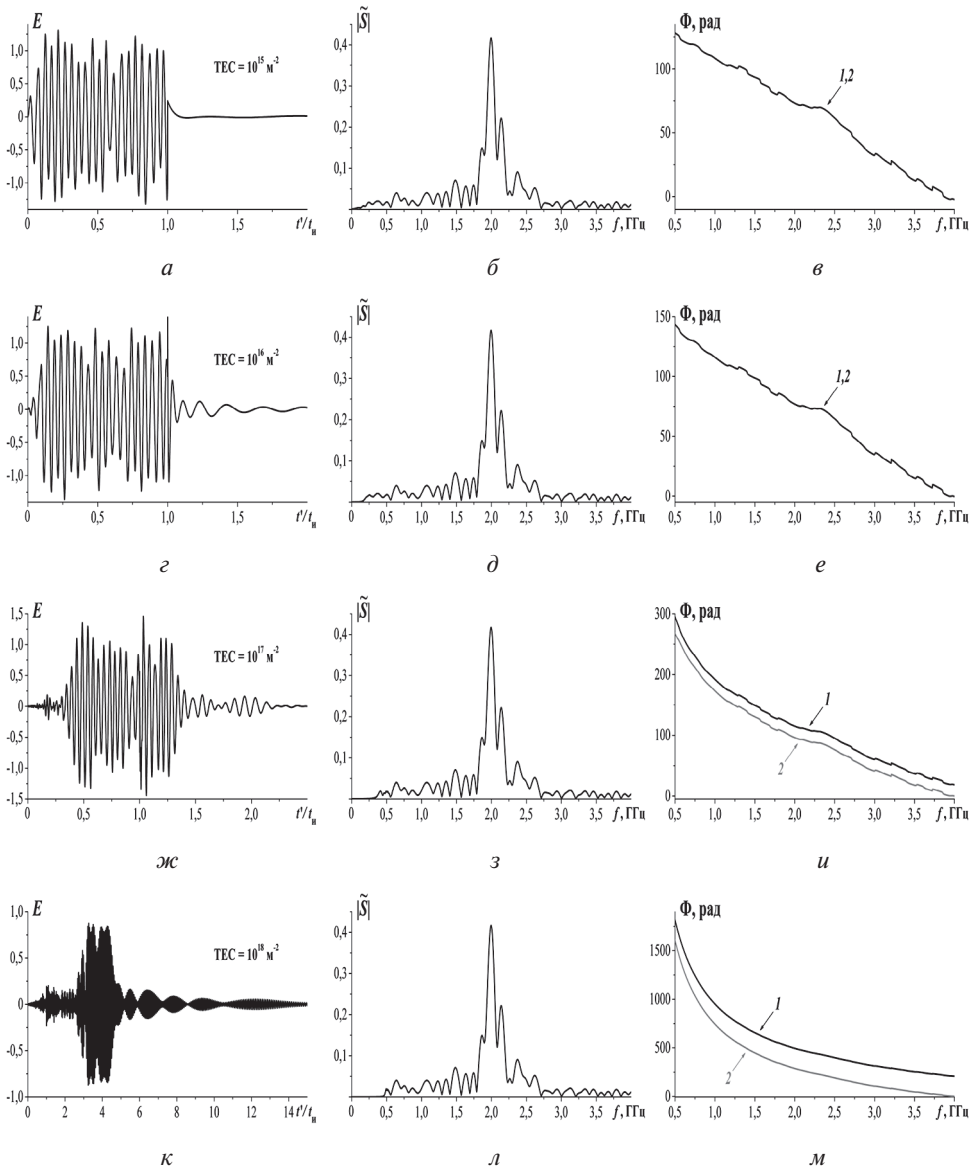
Рис. 5. То же, что и на рис. 3 для хаотического радиоимпульса (реализация 1), изображённого на рис. 1ж. \Phi = \Phi_{\text{изл}} + \Delta\Phi (в, е, и, м кривые 1); расчёт \Phi по деформированному импульсу (в, е, и, м кривые 2).
