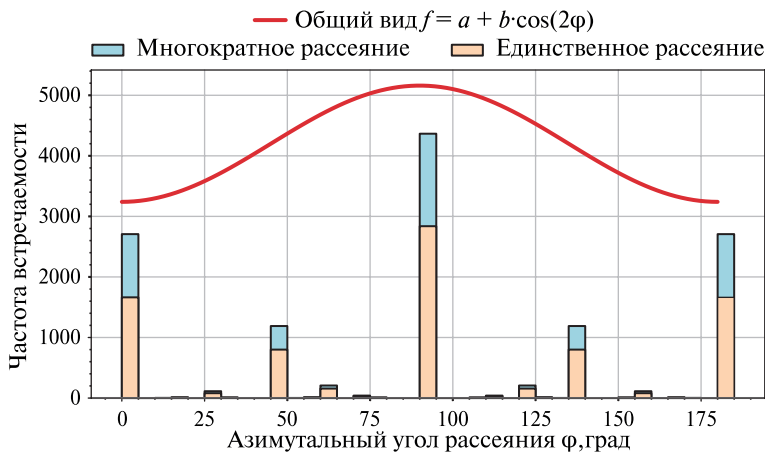
Рис. 4. Модуляционная кривая для СГС
