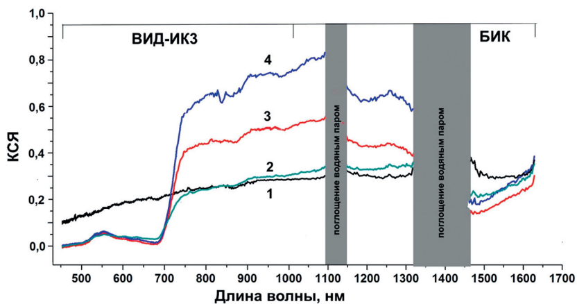
Рис. 17. Графики КСЯ для площадок 1–4 (см. рис. 10): 1 — асфальт; 2 — жухлая трава; 3 — зелёная трава; 4 — зелёные деревья
