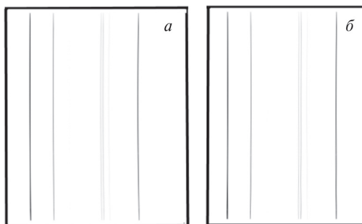
Рис. 9. Исправление дисторсии (распределение спектральной интенсивности линий ртутной лампы): a — исходное распределение; б — откорректированное распределение
