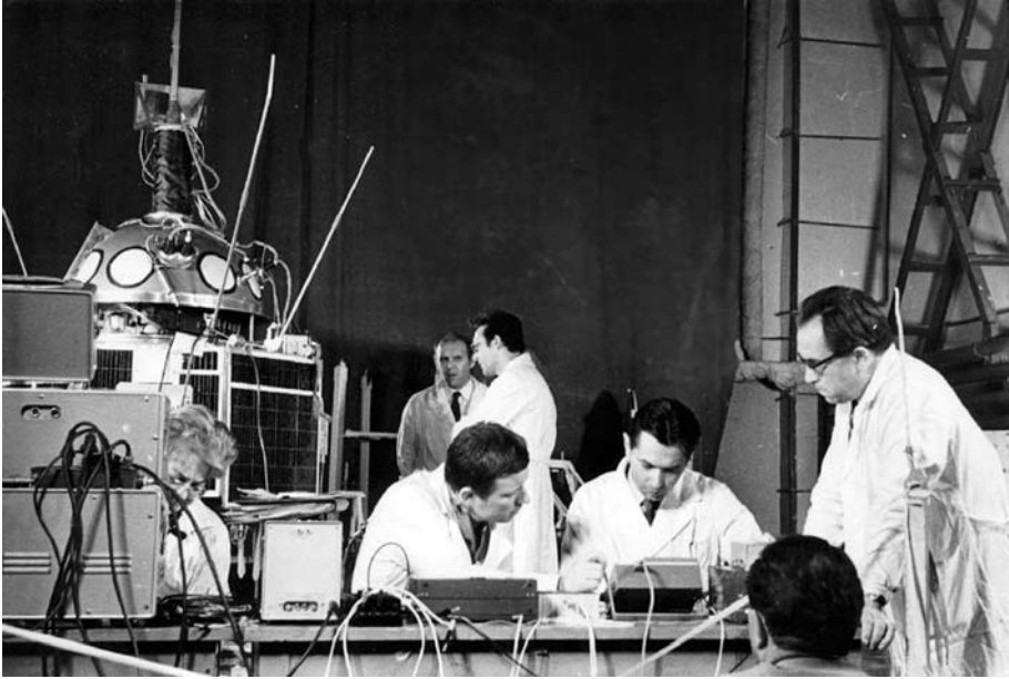
Испытания приборов и телеметрической системы ТС-1 на спутнике «Интеркосмос-5». За столом инженер Я. Войта, доктор П. Триска (ГФИ АН ЧССР), справа инженер В. Грим (институт TESLA VÜST), на заднем плане инженер К. Новотны (VZLÜ) и Л. Майер (институт TESLA VÜST). 1971 г.
