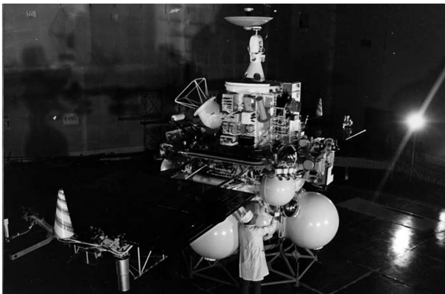
Космический аппарат «Фобос-1» в монтажно-испытательном корпусе космодрома Байконур, 1988 г.
