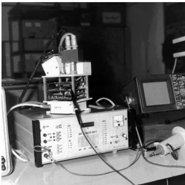
Рис. 6. Прибор VD-3 для проекта ФОБОС, 1982 г.
