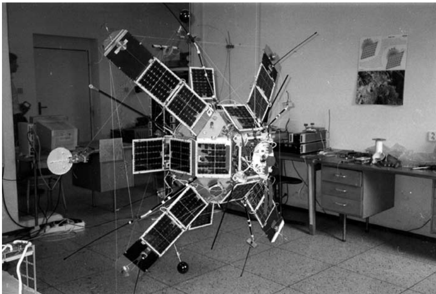
Спутник «Магيون-5» в летной конфигурации при измерении моментов инерции. Прага, ИФА АН ЧР, 1996 г.
