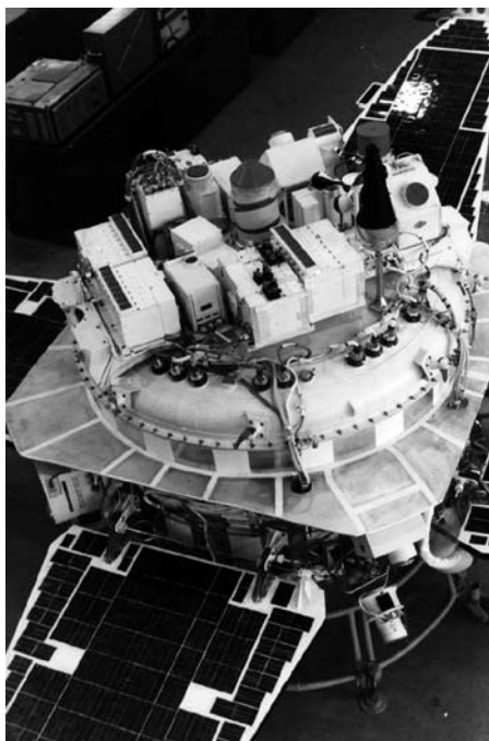
Рис. 4. КА «Прогноз-10» на заводе «Вымпел», 1985 г.
