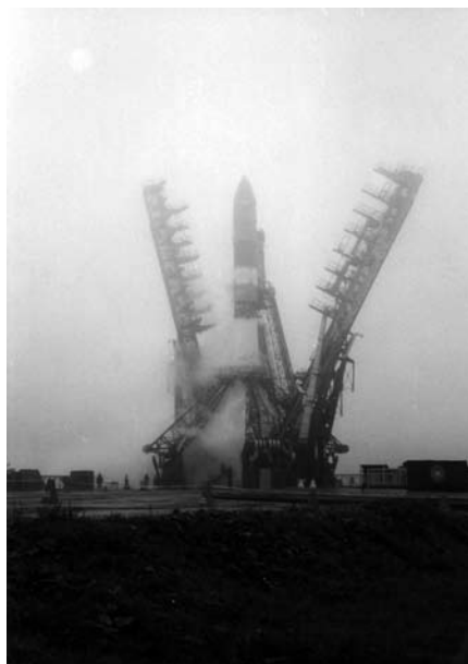
Отвод башни обслуживания, стартовый комплекс космодрома Плесецк, КА «Интербол-2», 1996 г.
