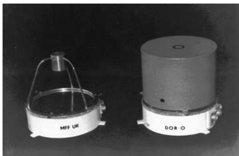
Рис. 3. Прибор ДОР для регистрации электронов высоких энергий
