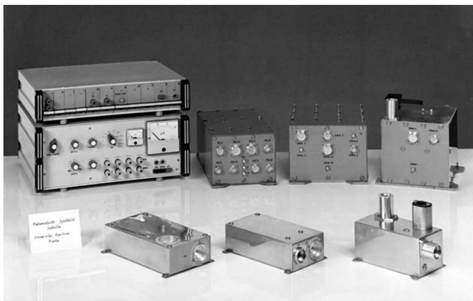
Рис. 2. Детекторы высокоэнергичных частиц прибора PG1-B (на переднем плане) и прибор ЕМА (справа сверху) для спутника «Интеркосмос-13», 1973 г.
