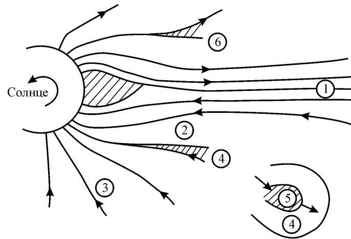
Рис. 6. Схематическое представление крупномасштабных типов солнечного ветра
