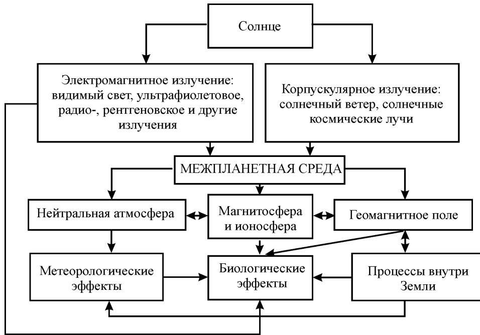
Рис. 1. Схема структуры солнечно-земных связей
