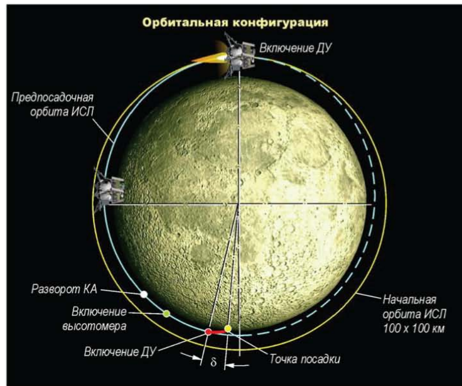
Рис. 2-2 Схема посадки
